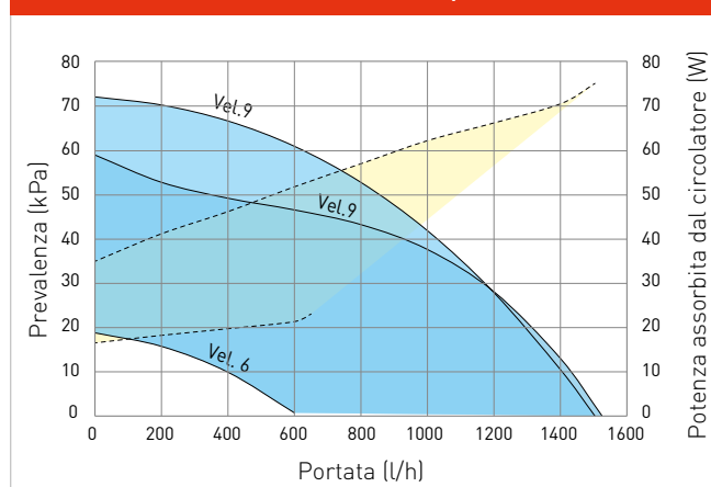
Grafico portata e prevalenza VICTRIX SUPERIOR 35/35 PLUS
